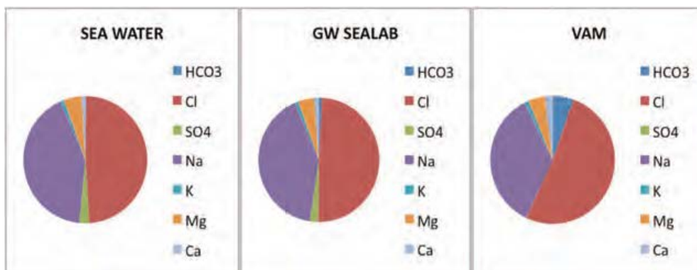
Figuur 3 Samenstelling (concentratie in mM) van zeewater en twee soorten grondwater (Uit: van der Hiele et al, 2014) waarvan de rechtersvariant niet geschikt was voor aquacultuur
