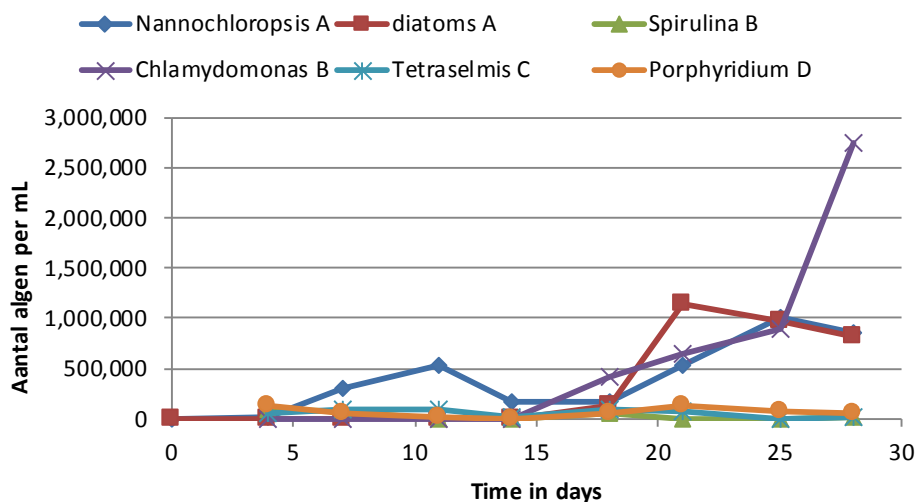
Figuur 11 Algengroei in 1 L reactoren in Test 5, gegroeid op 12,5x verdunde vloeibare fractie van digestaat. Hoofdletters At/m D geven de reactor weer
