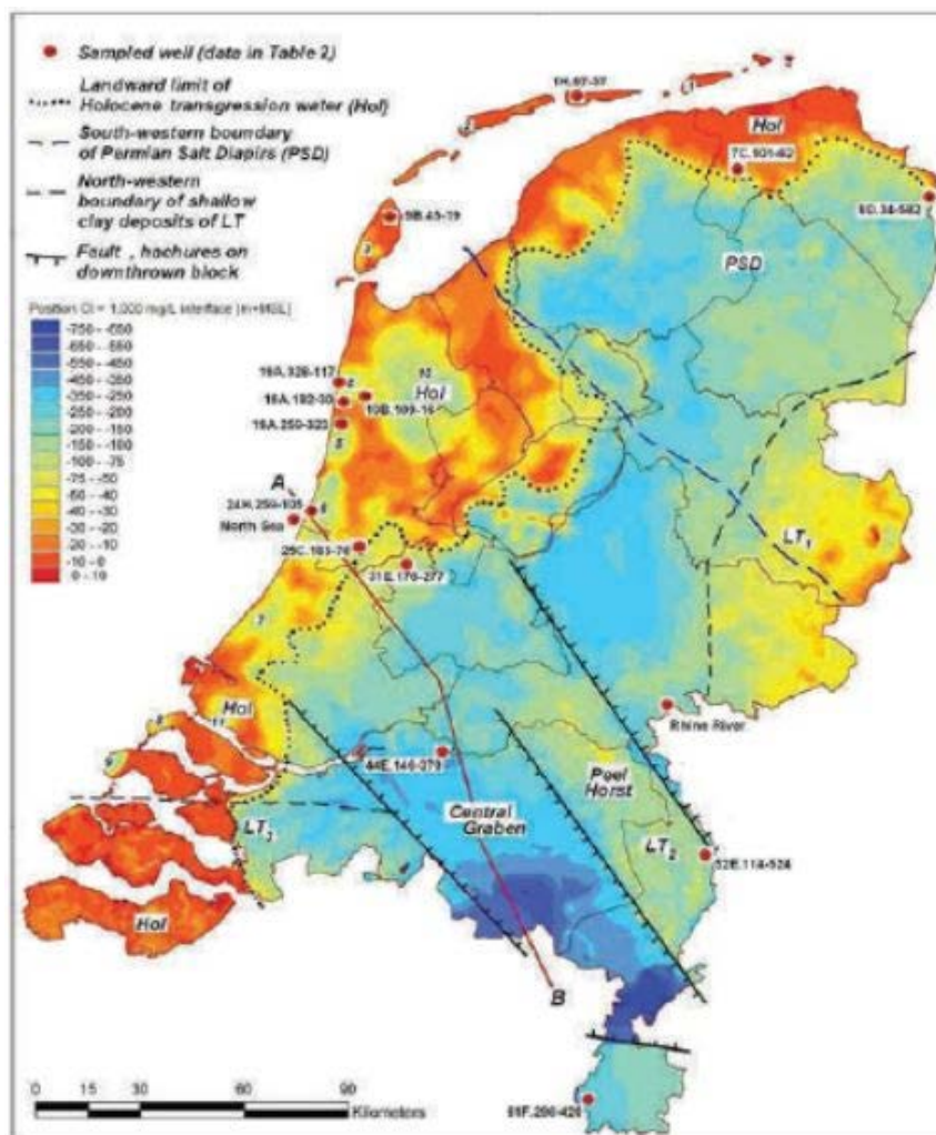
Figuur 2 Overzichtskaart van Nederland met diepte waarop zich de grens bevindt tussen zoet (<1 g Cl/L) en zout water (>1 g Cl/L). Rood geeft aan dat de grensvlak zich aan het maaiveld bevindt (zout grondwater), blauw geeft aan dat het grensvlak zich ver onder maaiveld bevindt (Uit: Stichting Waterbuffer, 2017)
